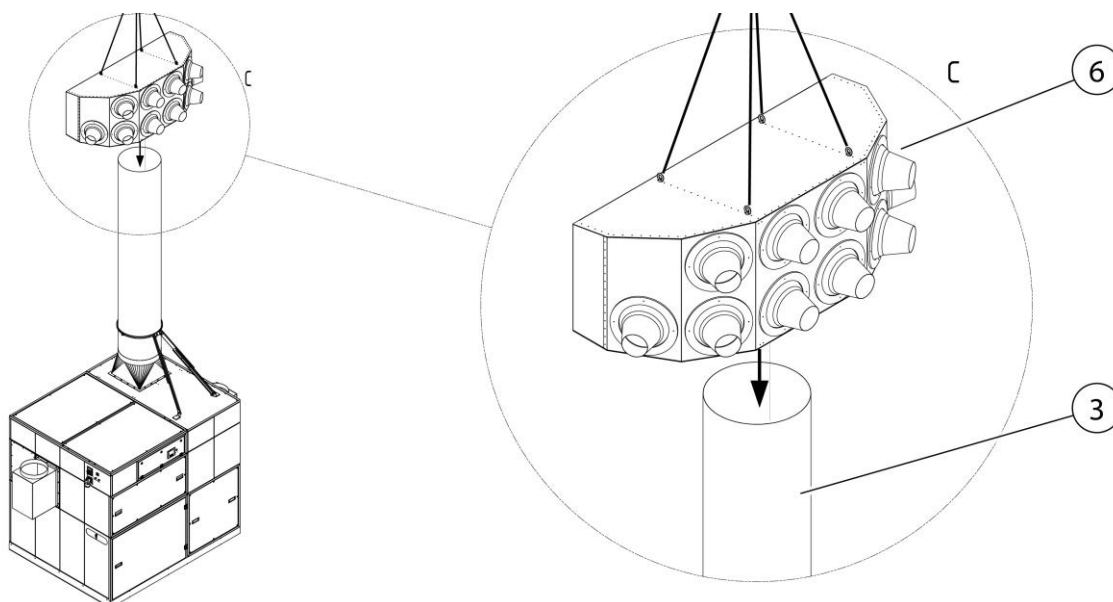
Obr. 13: Montáž vyfukovací jednotky
