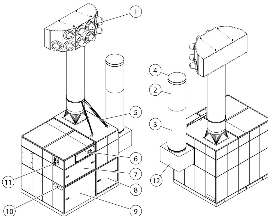
Obr. 6: Popis funkce – 998800463
