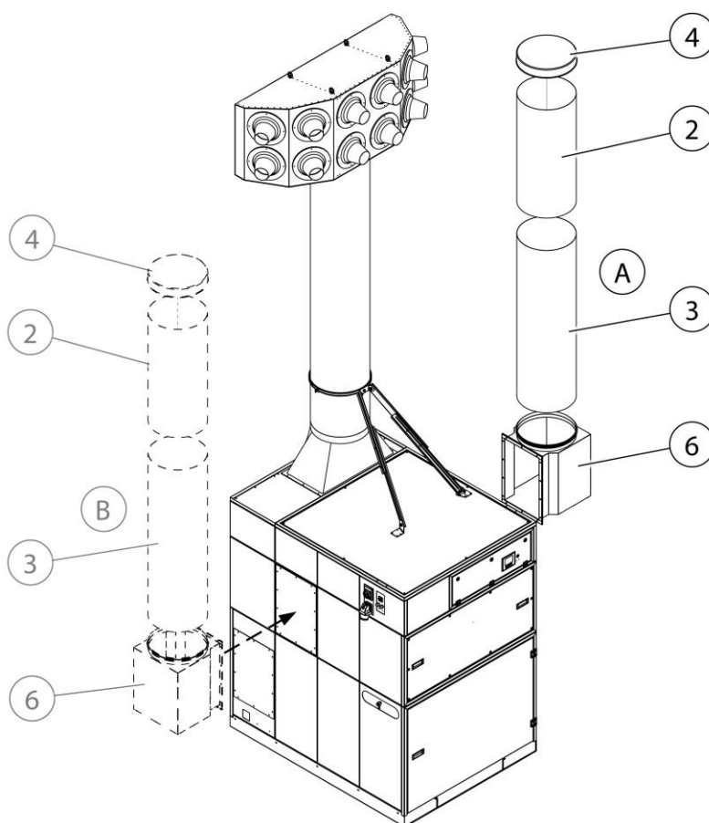
Obr. 16: Montáž sacího hrdla
