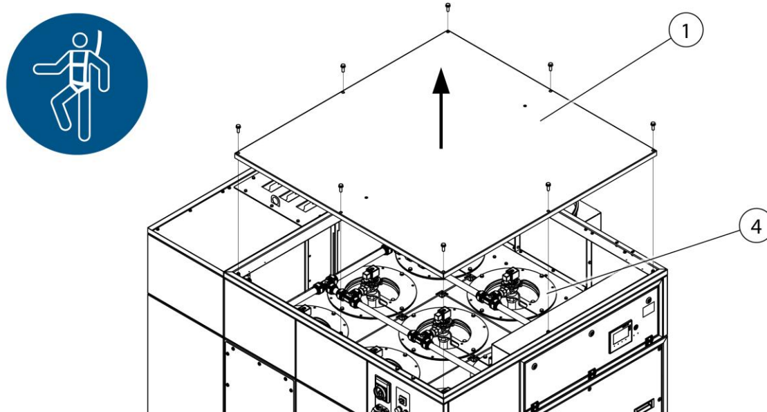
Obr. 42: Výměna filtru – demontáž filtračního plechu
