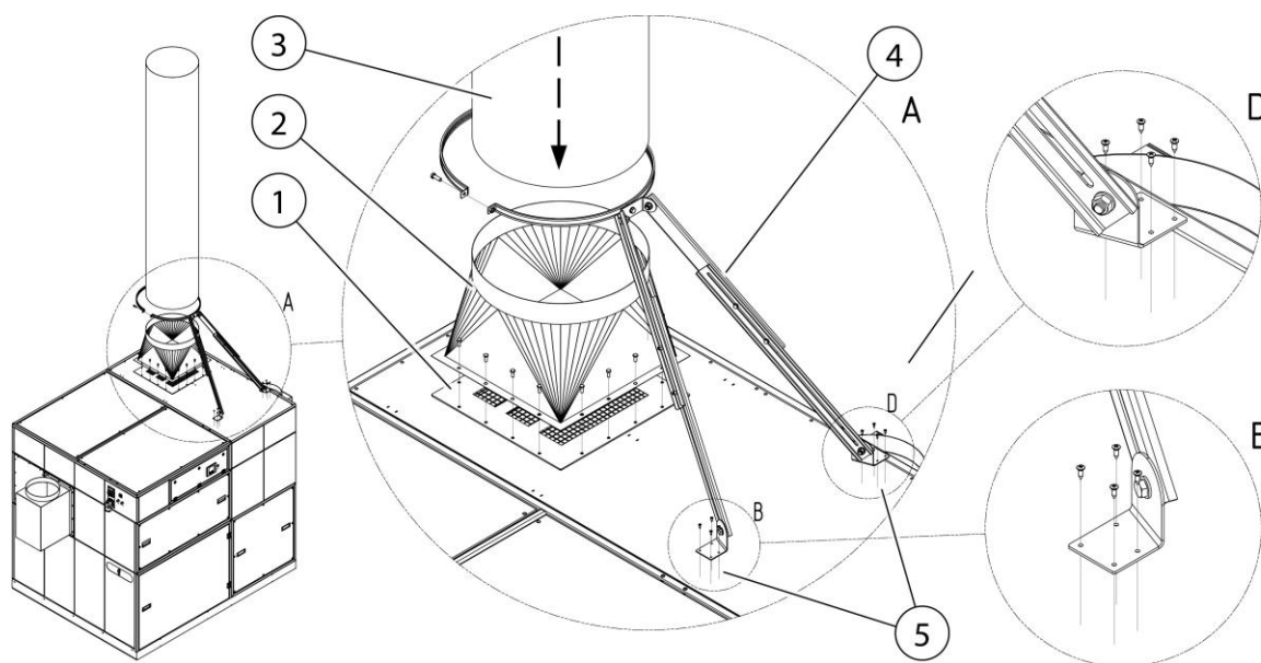
Obr. 12: Montáž vyfukovací jednotky
