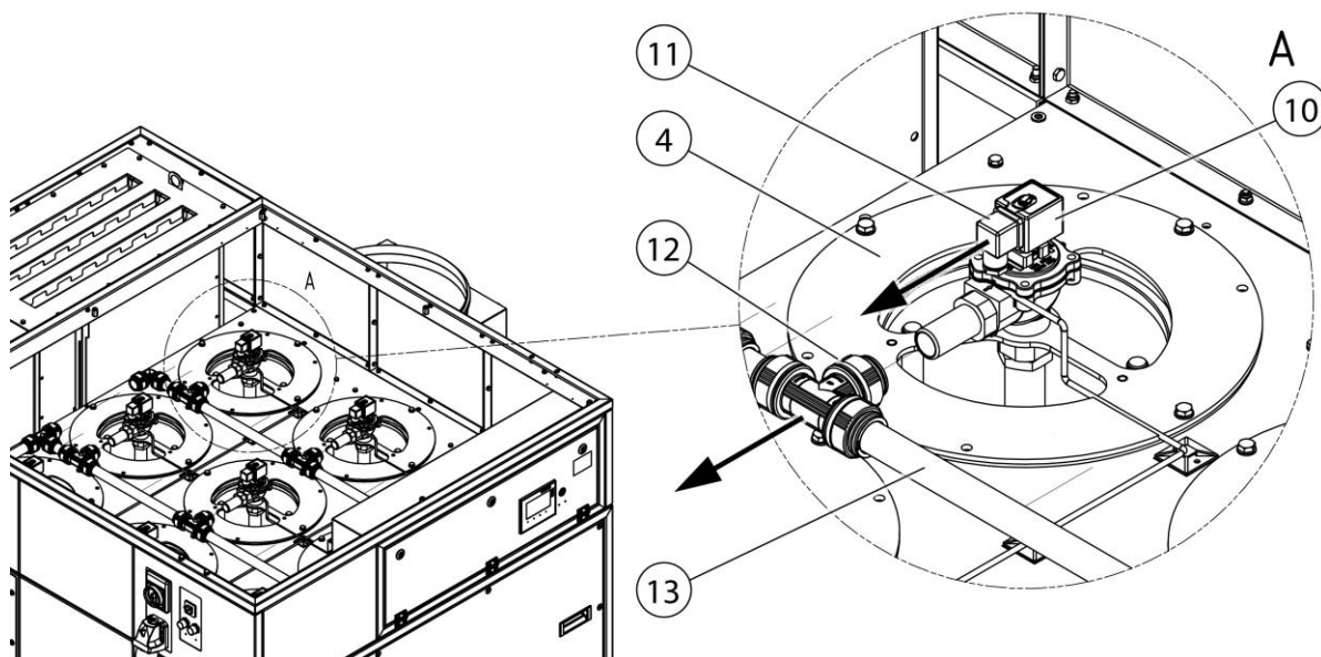
Obr. 43: Výměna filtru – demontáž připojení
