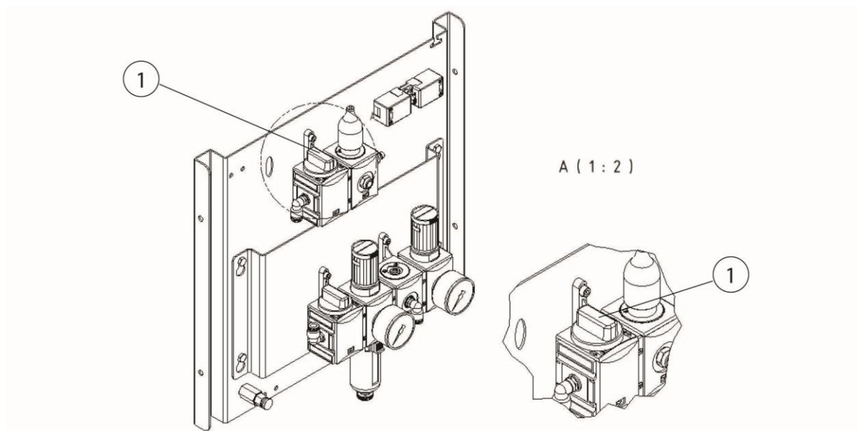
Obr. 34: Pneumatický ventil sběrné nádoby na prach
