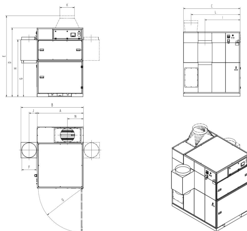
Obr. 55: Rozměrový výkres 998701371 (998800401, 998800462)
