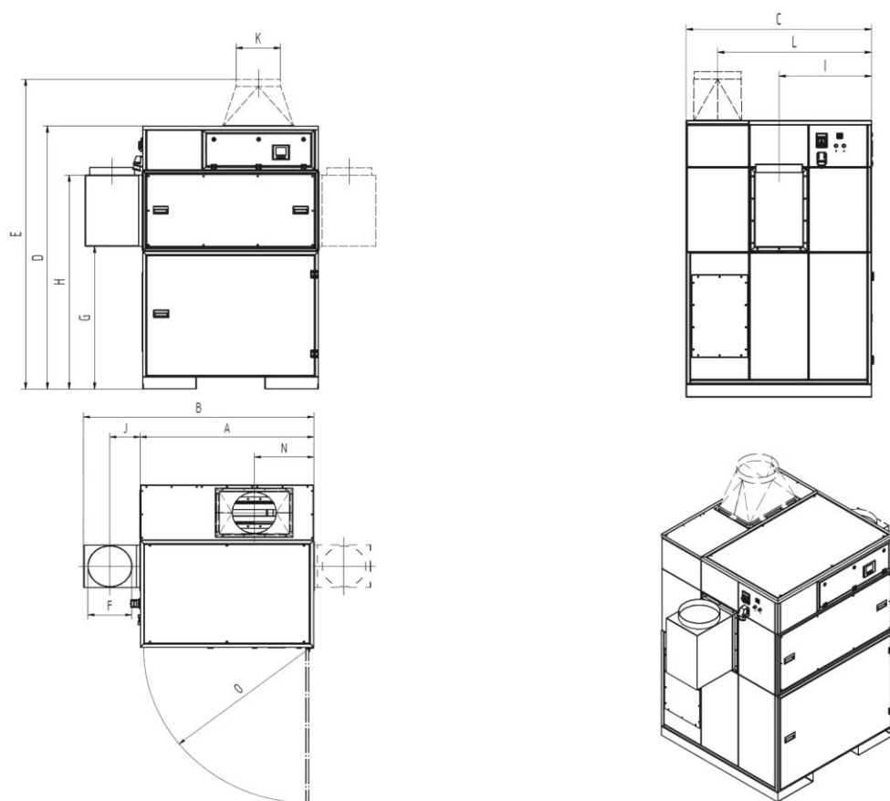
Obr. 54: Rozměrový výkres 998701372 (998800407, 998800461)
