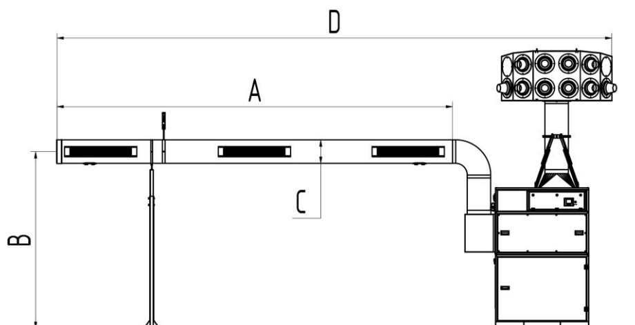
Obr. 57: Rozměrový výkres – 998800407
