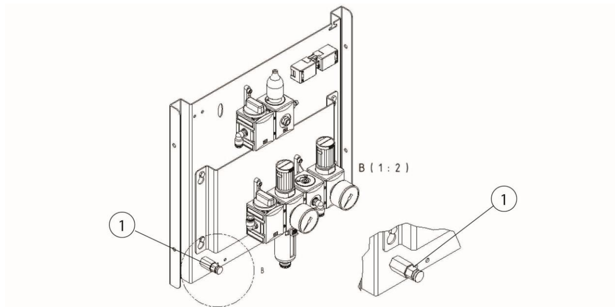
Obr. 48: Vypouštěcí ventil kondenzátu zásobníku stlačeného vzduchu
