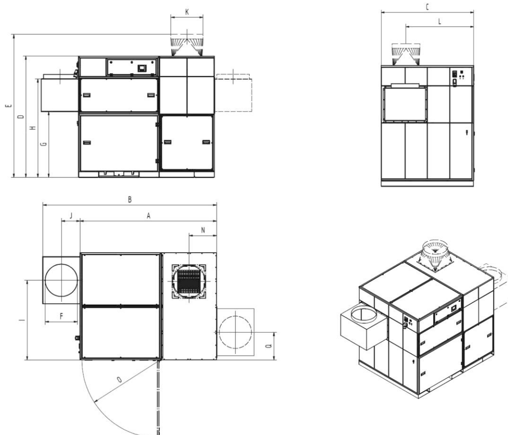
Obr. 56: Rozměrový výkres 998701370 (998800414, 998800463)
