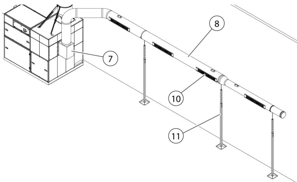
Obr. 15: Montáž na zem – sací potrubí
