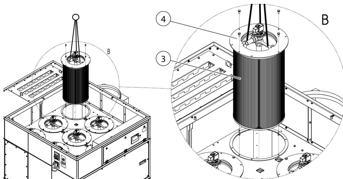
Obr. 45: Výměna filtru – demontujte držák filtru
