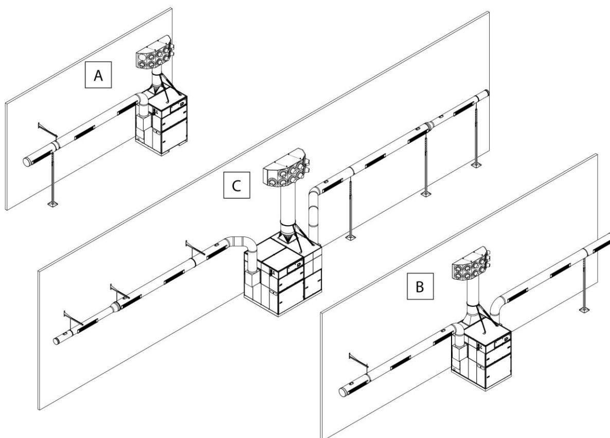
Obr. 11: Montáž – přehled variant produktů
