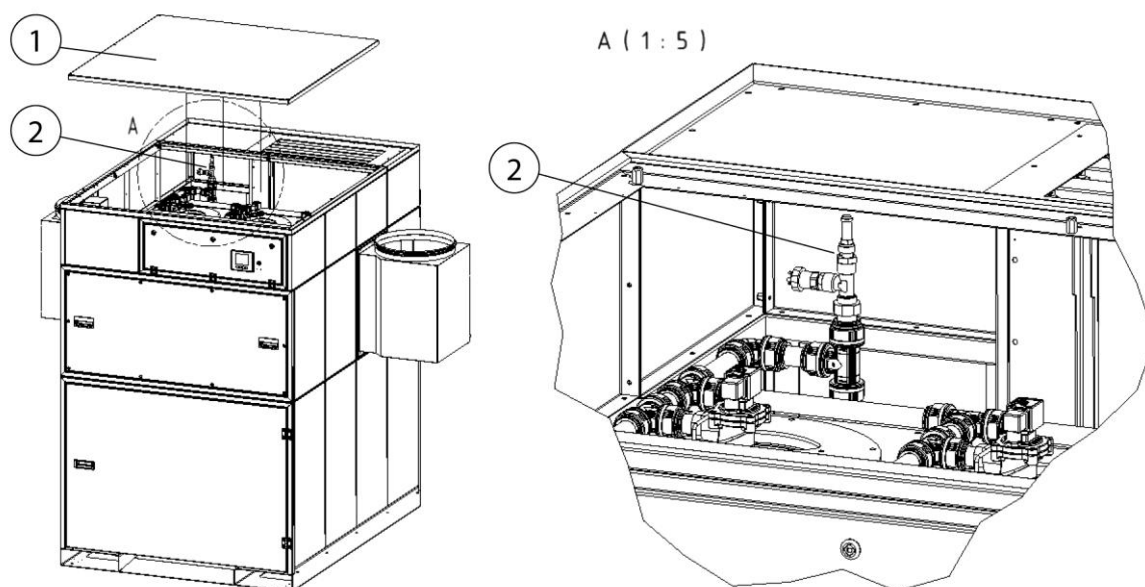
Obr. 53: Přístup k pneumatickému pojistnému ventilu
